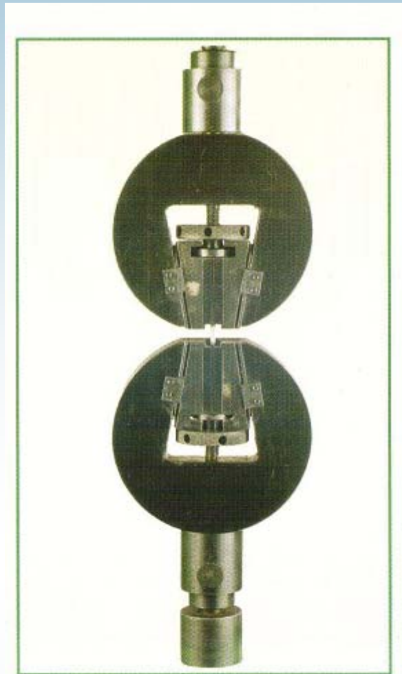
Vice cum Wedge Type Grip
